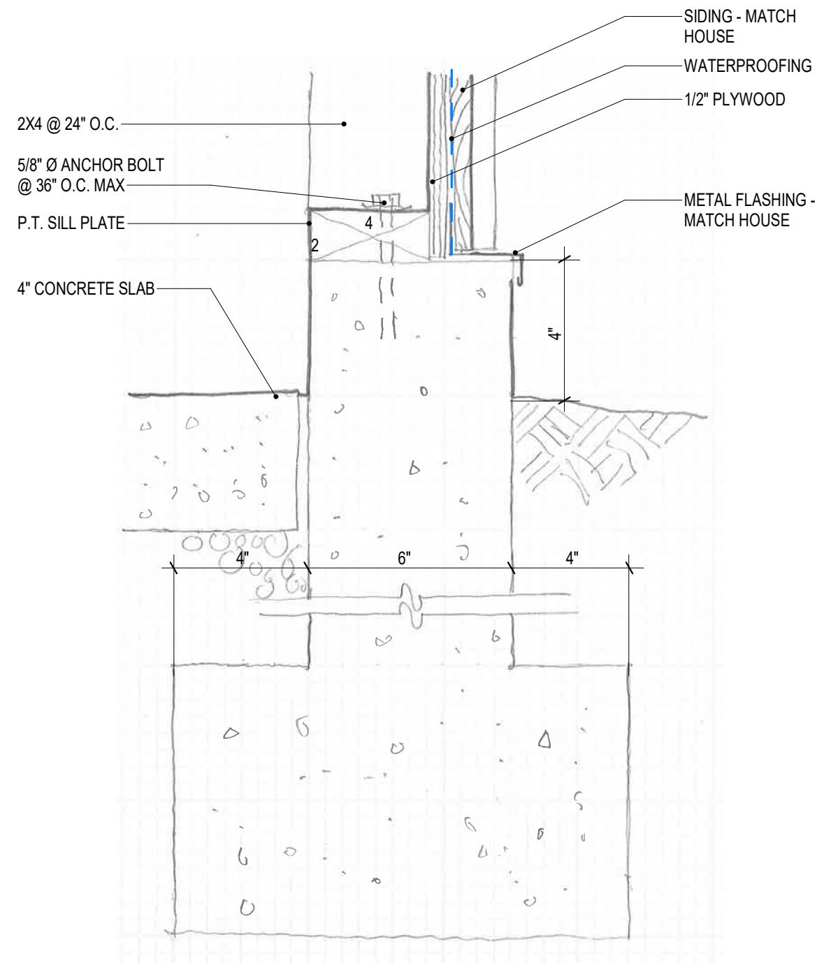
Detail 3.0 SCALE: 12" = 1'-0"
