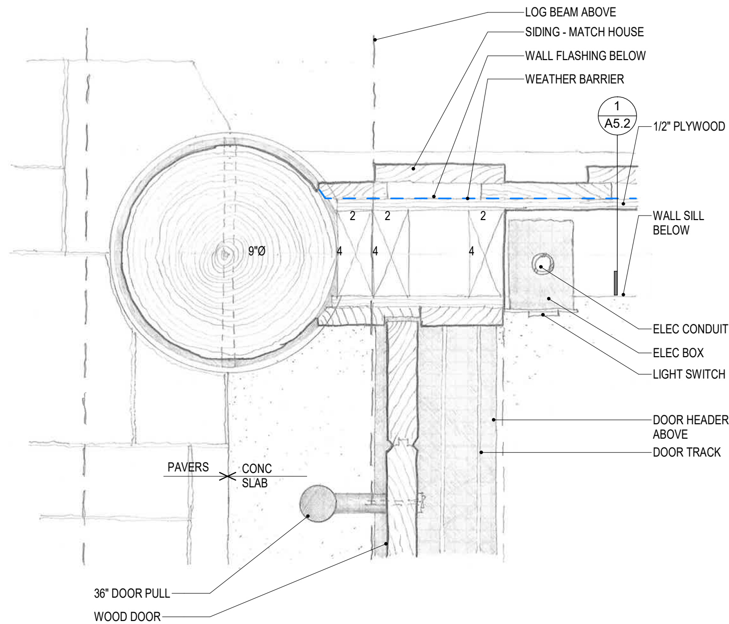
Detail 2.0 SCALE: 12" = 1'-0"
